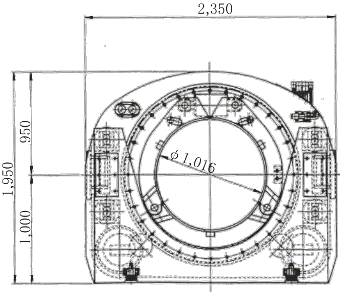
正面图
