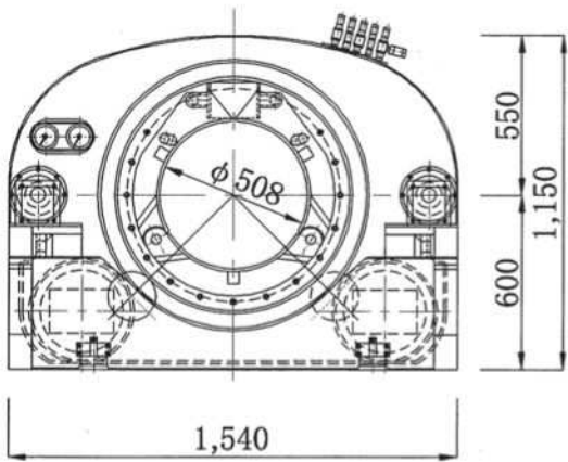
正面图
