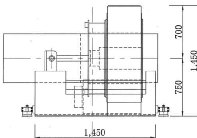
侧面图
