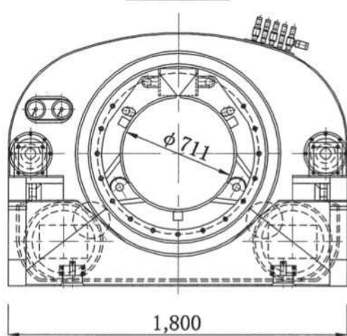
正面图
