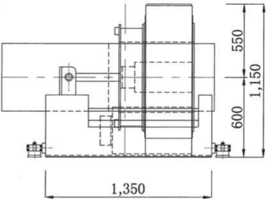
侧面图
