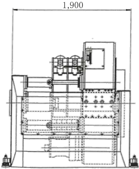
侧面图
